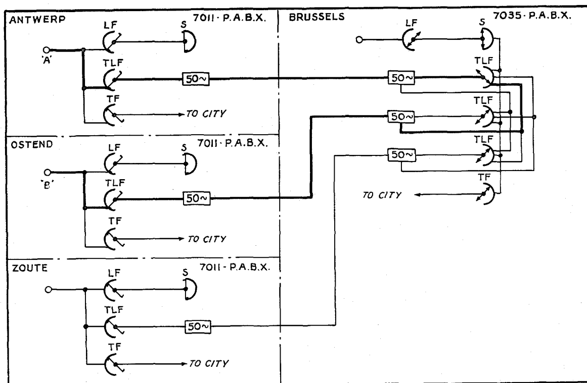
Fig. 2—Function Diagram.
